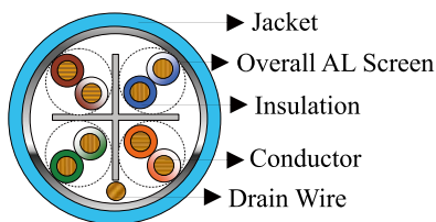
Cat6 F/UTP
