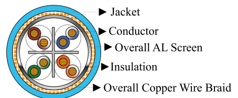
Cat6 S/FTP
