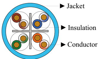
Cat6 U/UTP
