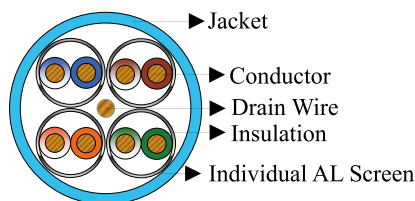
Cat6 U/FTP
